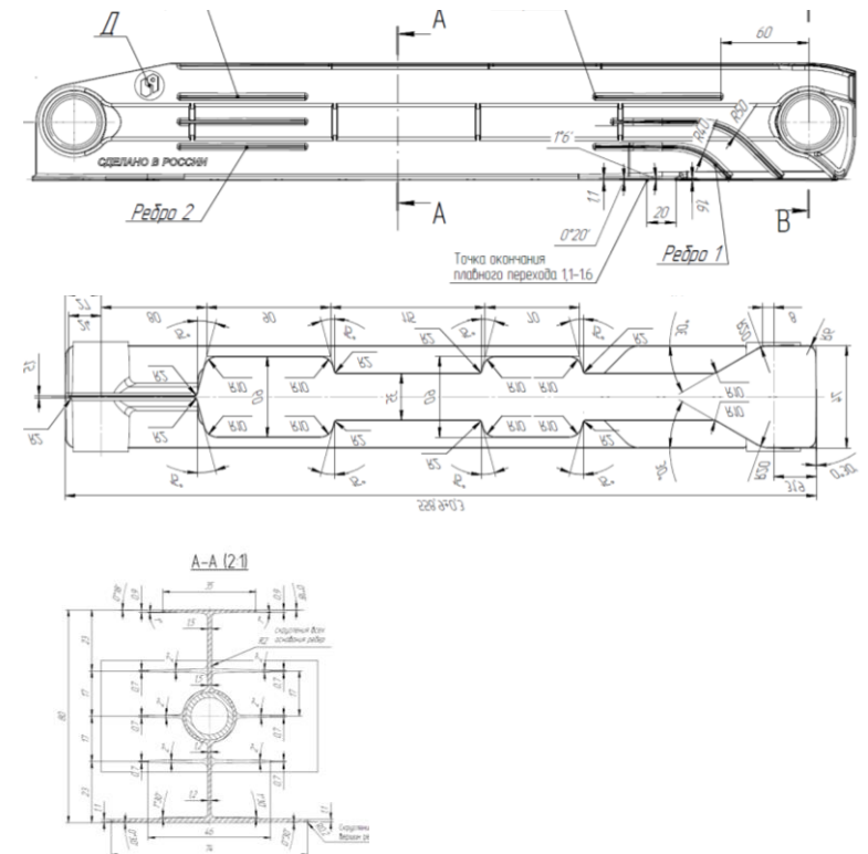
Схема радиатора Корвет BM и AL 500x100 облегчённая модель
