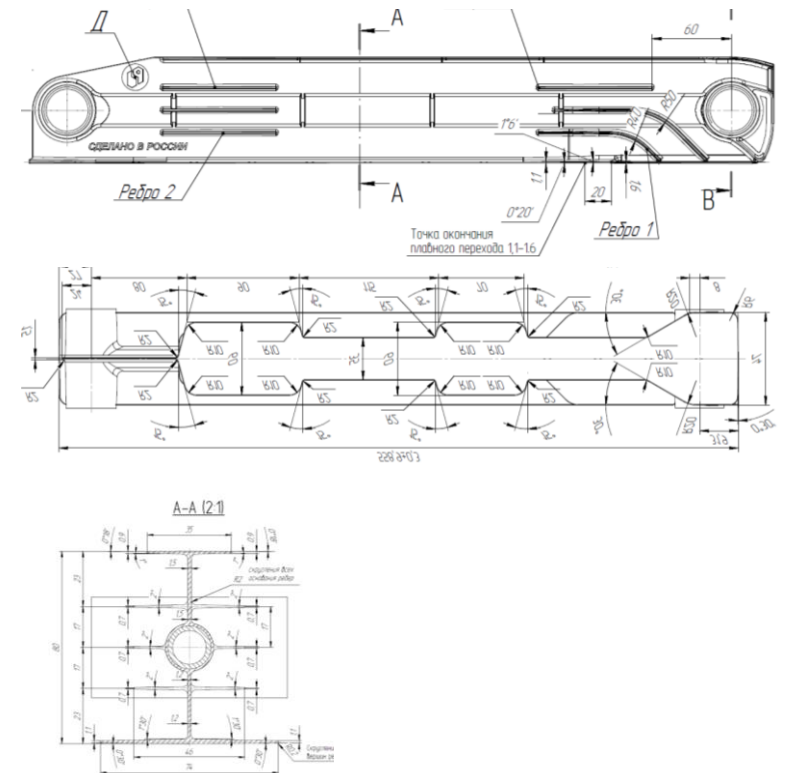
Схема радиатора Корвет ВМ и АL 500x100 облегчённая модель
